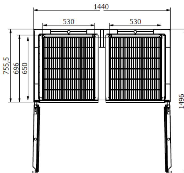
Vue de haut porte ouverte
